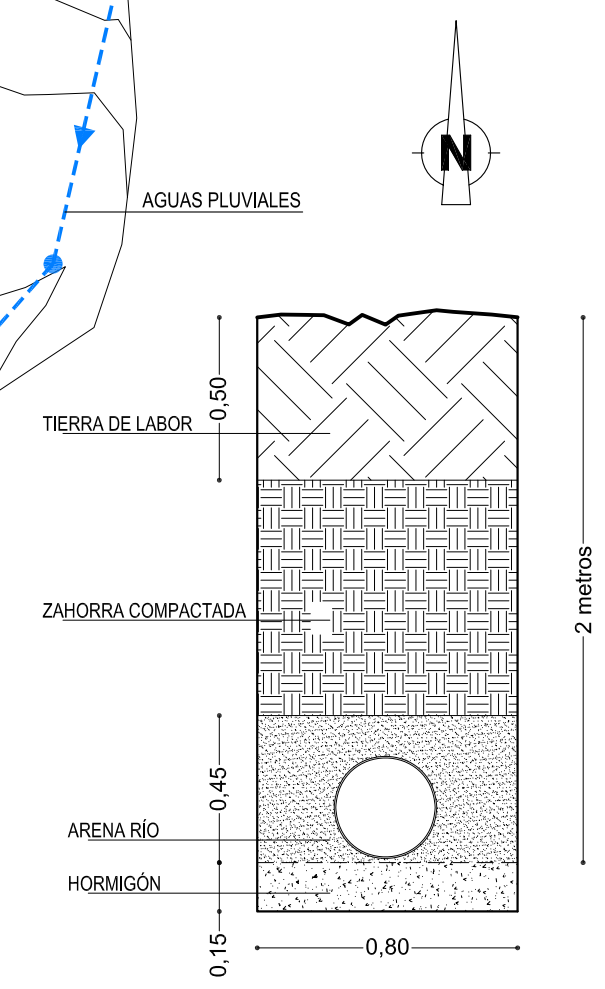
Detalle de zanja tipo para colector que atraviesa los campos de cultivo
